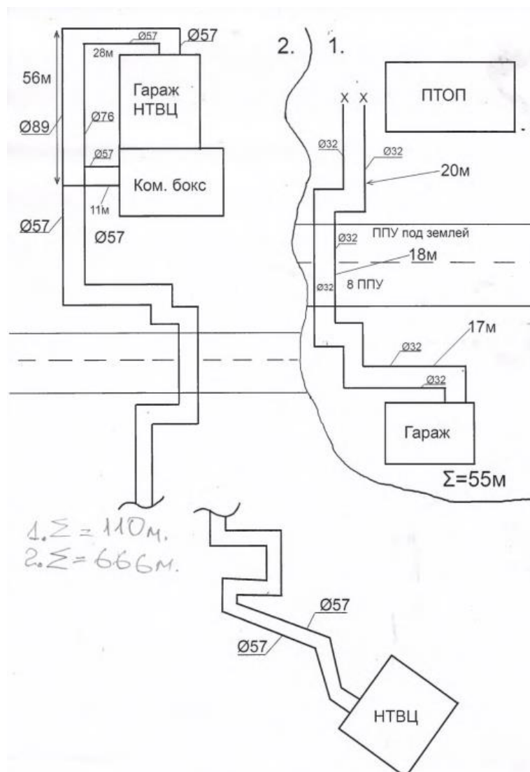
Рисунок 2 – Схема тепловых сетей (реконструкция)
