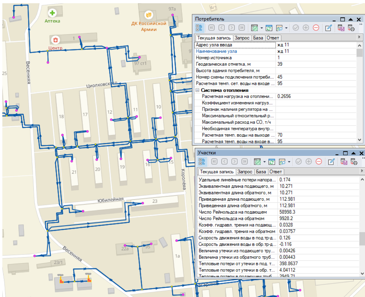
Рисунок 1 - Графическое представление электронной модели
